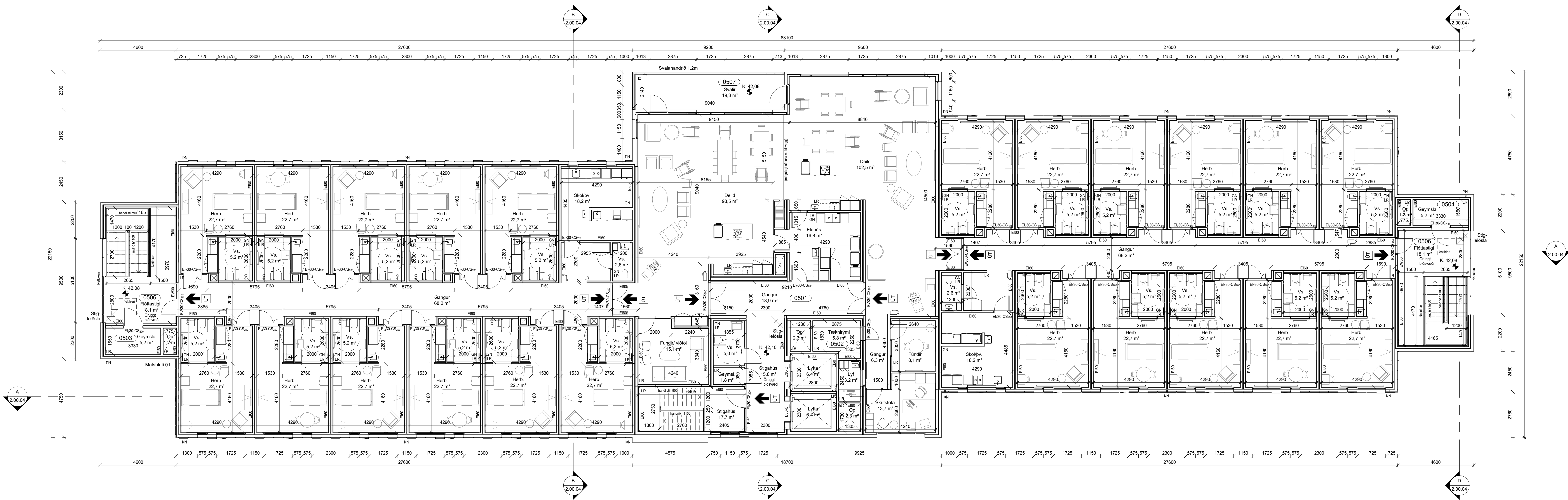
5 GRUNNMYND 5. HÆÐ 1 : 100
