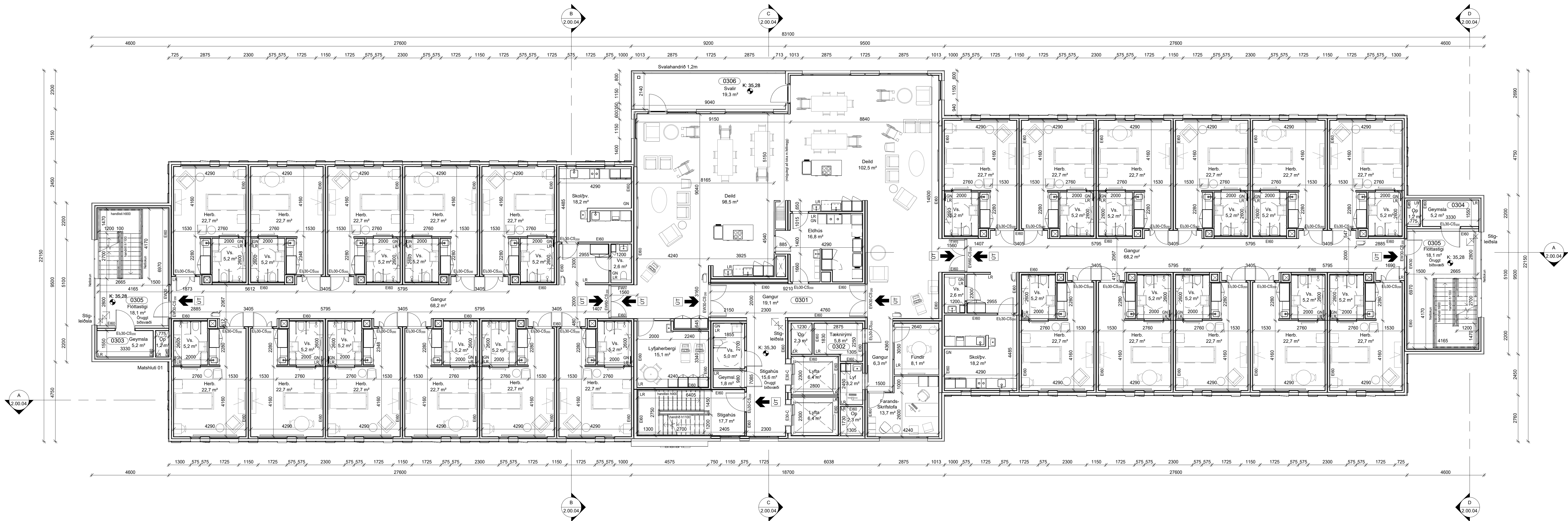
3 GRUNNMYND 3. HÆÐ 1:100
