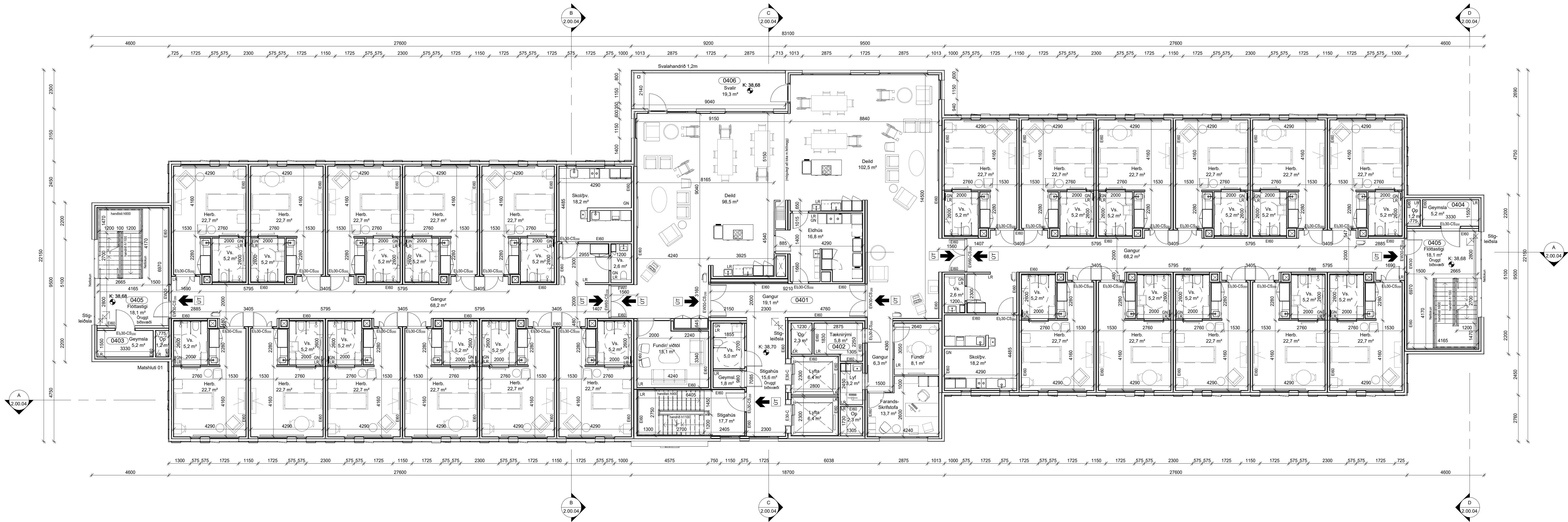
4 GRUNNMYND 4. HÆÐ 1:100
