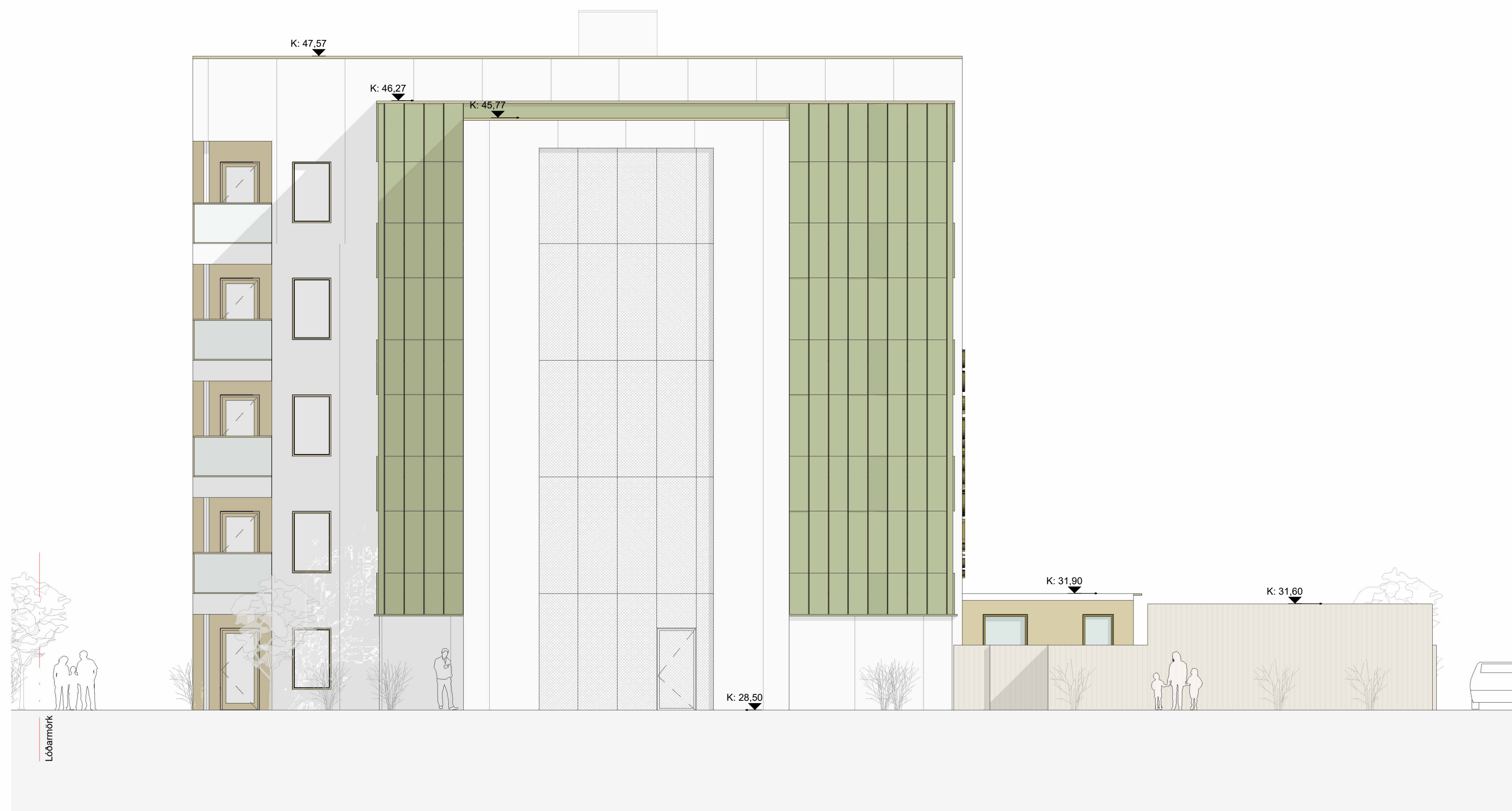
S ÁSÝND - SUÐURHLIÐ 1 : 100
