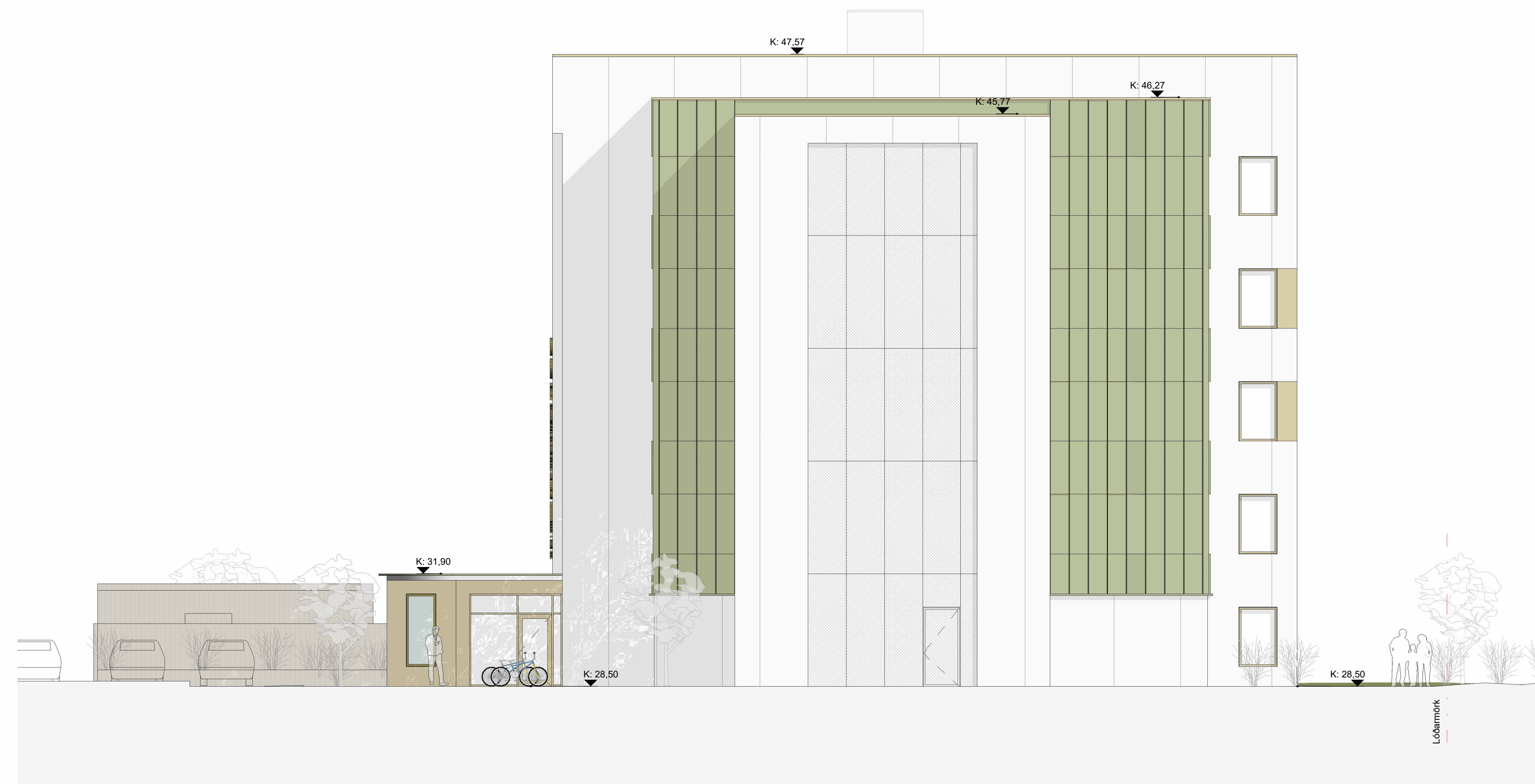
N ÁSÝND - NORÐURHLIÐ 1 : 100
